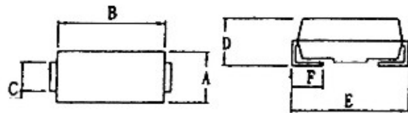
DIMENSION 尺寸
