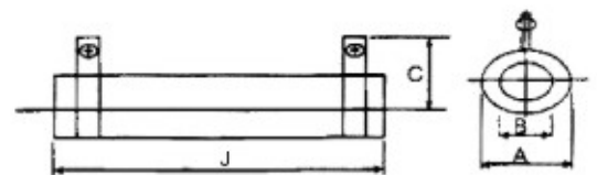
波浪型 RIBBON WIREWOUND RESISTOR
