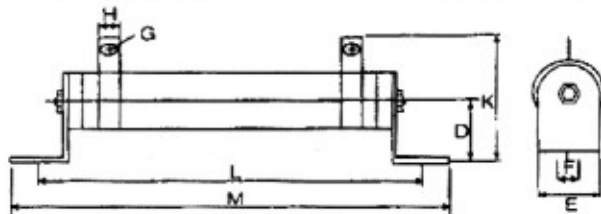
平面繞線型 PLATE RESISTOR
